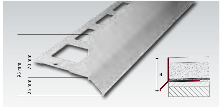
Kiesbettprofile aus Aluminium, gestanz, Auflageschenkel: 100 mm
