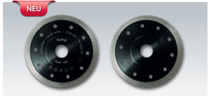
High-End-Diamantscheiben, Ø 125 mm, 1,3 mm dünn, Ornamentsegment, verstärkter Flansch
