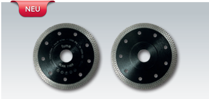
High-End-Diamantscheiben, Ø 115 mm, 1,3 mm dünn, Ornamentsegment, verstärkter Flansch
