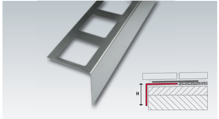
Balkonabdeckprofile aus Edelstahl, Oberfläche: Pulverbeschichtung , Auflegeschenkel: 80 mm
