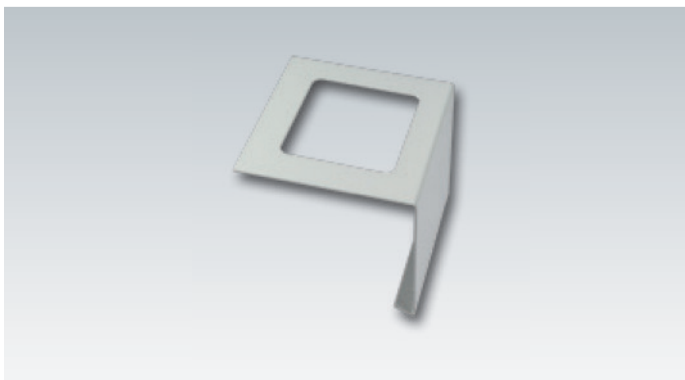
Verbinder für Balkonabdeckprofile, gestanz, Oberfläche: Pulverbeschichtung , Auflegeschenkel: 80 mm
