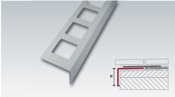
Balkonabdeckprofile aus Aluminium, gestanz, Oberfläche: Pulverbeschichtung , Auflegeschenkel: 80 mm
